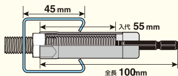
浅型チャンネル用 No. KAR201710
