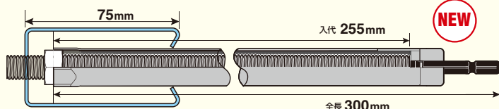
深型チャンネル用 No. KAR201730
