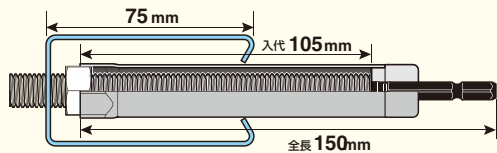
深型チャンネル用 No. KAR201715
